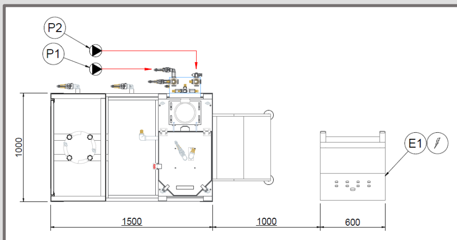
Vista dall'alto
